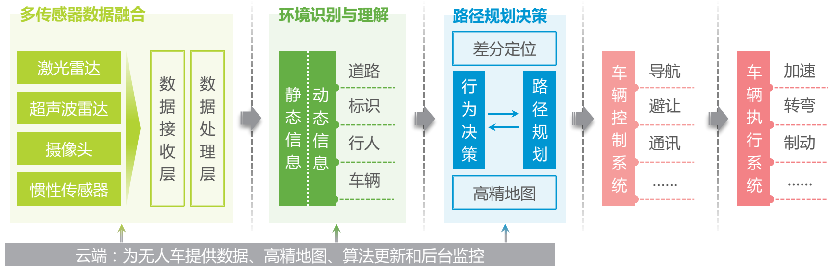
无人配送车自动驾驶系统流程示意图
